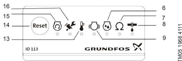
Рис. 126 Индикаторы на модуле IO 113
