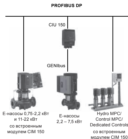
Рис. 132 Модуль CIM/CIU 150 в сети PROFIBUS
