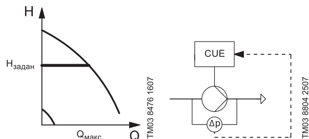
Рис. 64 Постоянный перепад давления насоса
