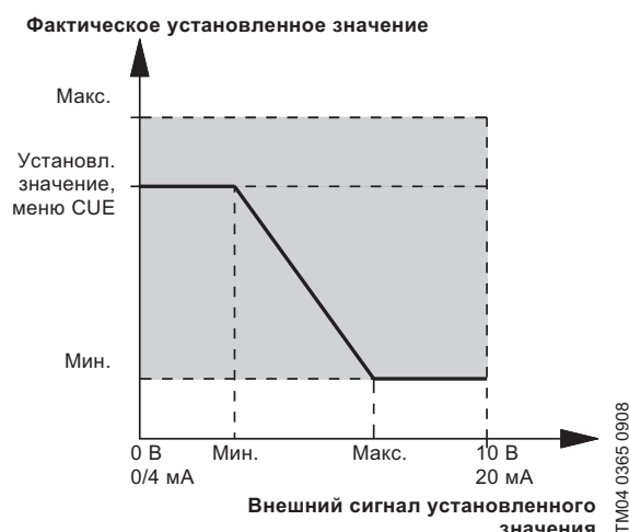
Рис. 77 Сокращённый обратный внешний сигнал установленного значения
