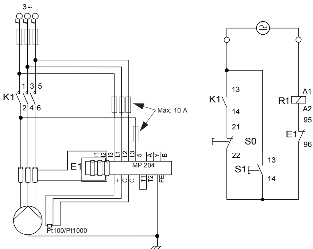
Рис. 121 Трёхфазное соединение с трансформаторами тока
