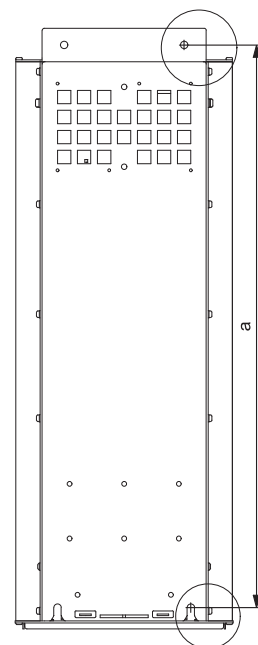
Рис. 107 Корпуса A4, A5, B1, B2, B3, B4, C1, C2, C3 и C4
