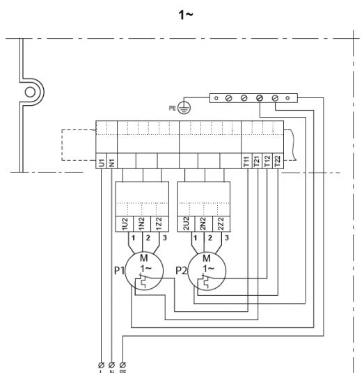
Схема подключения двух однофазных насосов без встроенных конденсаторов.
