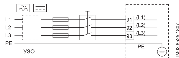
Рис. 96 Пример подключения CUE к трёхфазной сети с сетевым выключателем, плавкими предохранителями и дополнительной защитой
