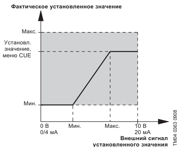
Рис. 75 Сокращённый внешний сигнал установленного значения
