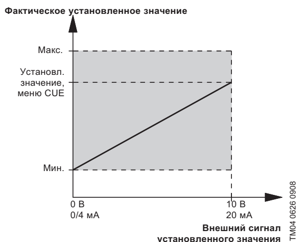
Рис. 74 Внешнее установленное значение
