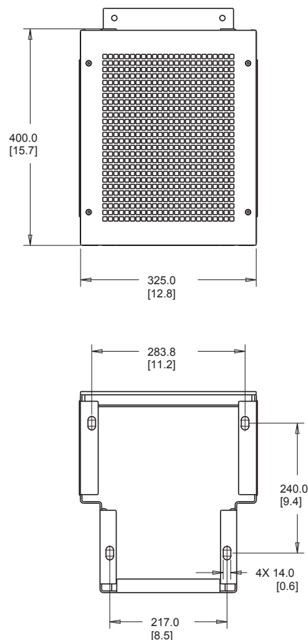
Рис. 115 Шаблон для сверления под цоколь D1h (мм)
