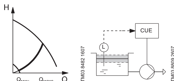
Рис. 69 Постоянный уровень с функцией останова
