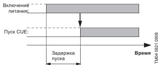
Рис. 92 Задержка пуска после включения питания
