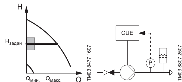
Рис. 67 Постоянное давление с функцией останова
