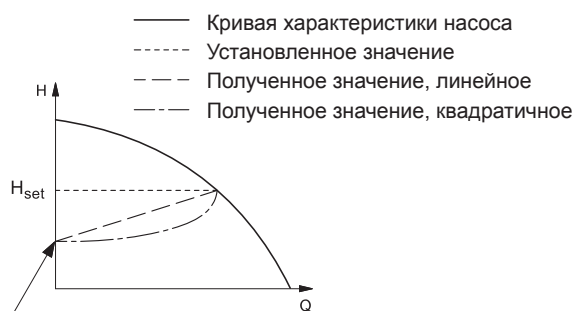
Рис. 34 Пропорциональное регулирование давления
