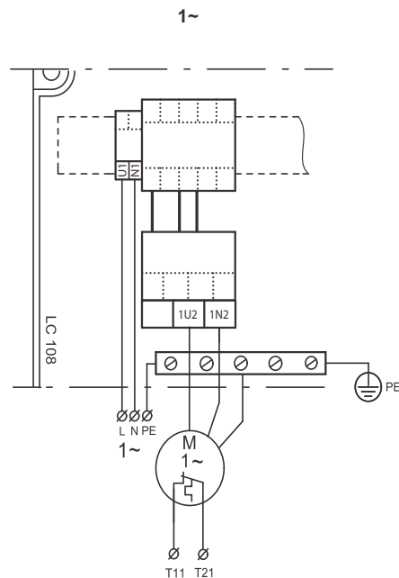
Схема подключения однофазного насоса со встроенным конденсатором
