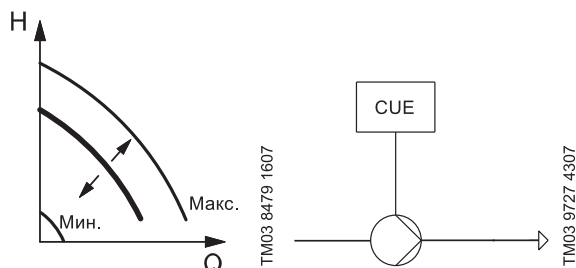
Рис. 62 Разомкнутый контур, постоянная характеристика
