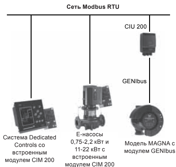
Рис. 134 Модуль CIM/CIU 200 в сети Modbus
