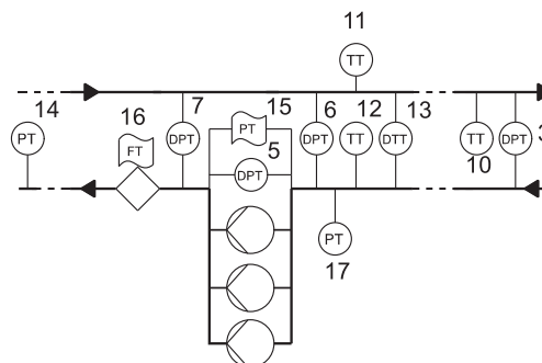
Рис. 32 Отопление и охлаждение, насосы в обратном трубопроводе
