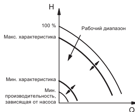
Рис. 86 Рабочий диапазон CUE
