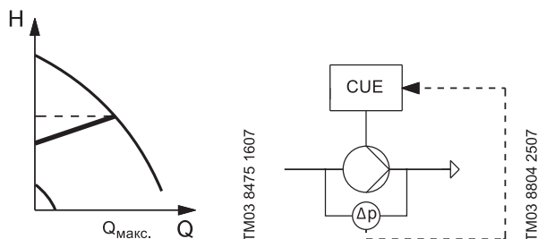
Рис. 63 Пропорциональный перепад давления
