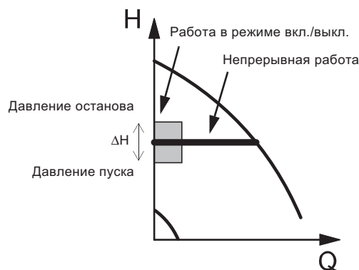
Рис. 81 Постоянное давление с функцией останова. Разница между значениями давления срабатывания на пуск и останов насоса ( \Delta H )
