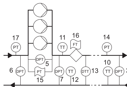
Рис. 31 Отопление и охлаждение, насосы в подающем трубопроводе
