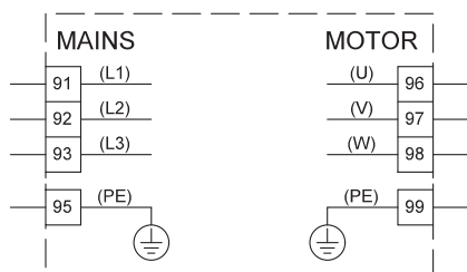
Рис. 97 Схема соединений, подключение к сети трёхфазного тока
