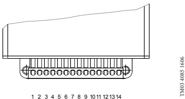
Рис. 128 Соединительные контакты
