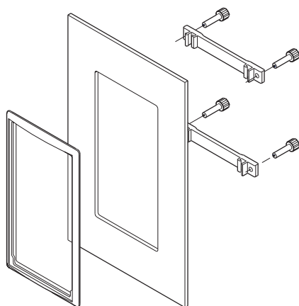
Рис. 113 Комплект для монтажа GLCP на расстоянии
