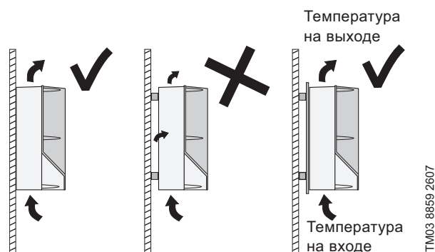
Рис. 94 Вешайте устройство CUE непосредственно на стену или устанавливайте на пластину
