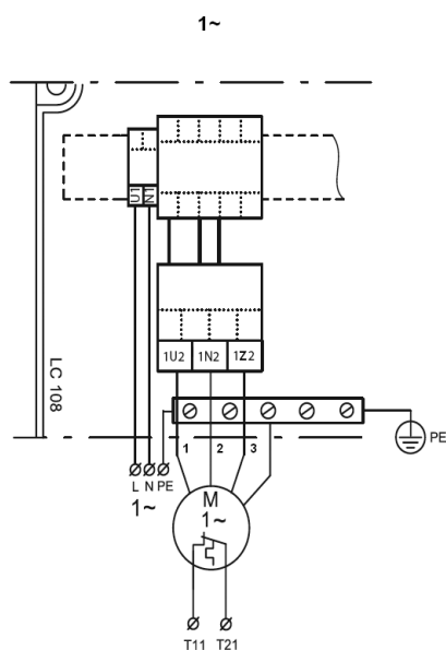
Схема для подключения однофазного насоса без встроенных конденсаторов.
