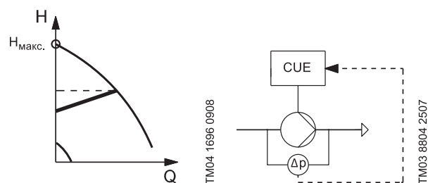
Рис. 90 Пропорциональный перепад давления, обновление H_{\text{макс}}
