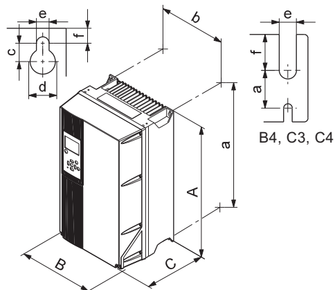
Рис. 107 Корпуса A4, A5, B1, B2, B3, B4, C1, C2, C3 и C4
