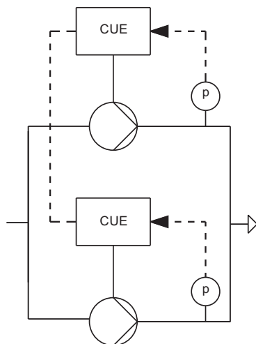
Рис. 85 Два насоса, соединённых параллельно и регулируемых через GENIbus
