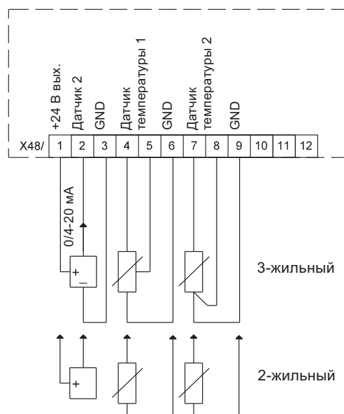
Рис. 111 Схема электрических соединений, MCB 114
