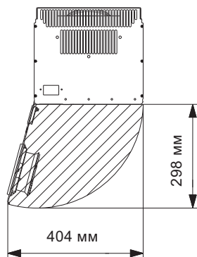
Рис. 95 Свободное пространство перед CUE, корпус D1h и D2h
