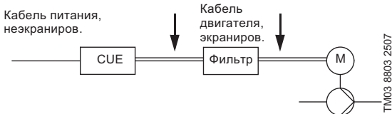
Рис. 100 Пример монтажа с фильтром. Кабель между CUE и фильтром должен быть коротким
