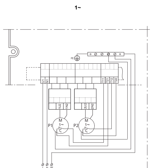
Схема подключения двух однофазных насосов со встроенным конденсатором.
