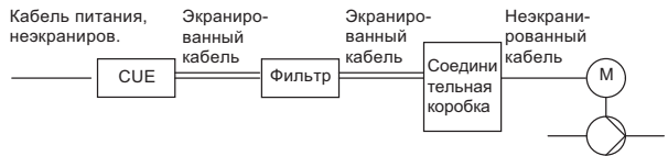
Рис. 102 CUE и фильтр установлены на расстоянии от скважины. Панель управления
