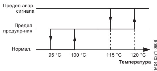
Рис. 87 Контроль температуры подшипников с использованием предельных значений для предупреждений и аварийных сигналов
