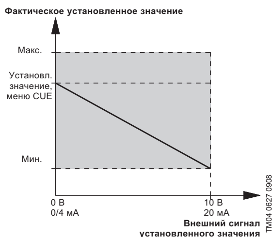
Рис. 76 Обратный внешний сигнал установленного значения
