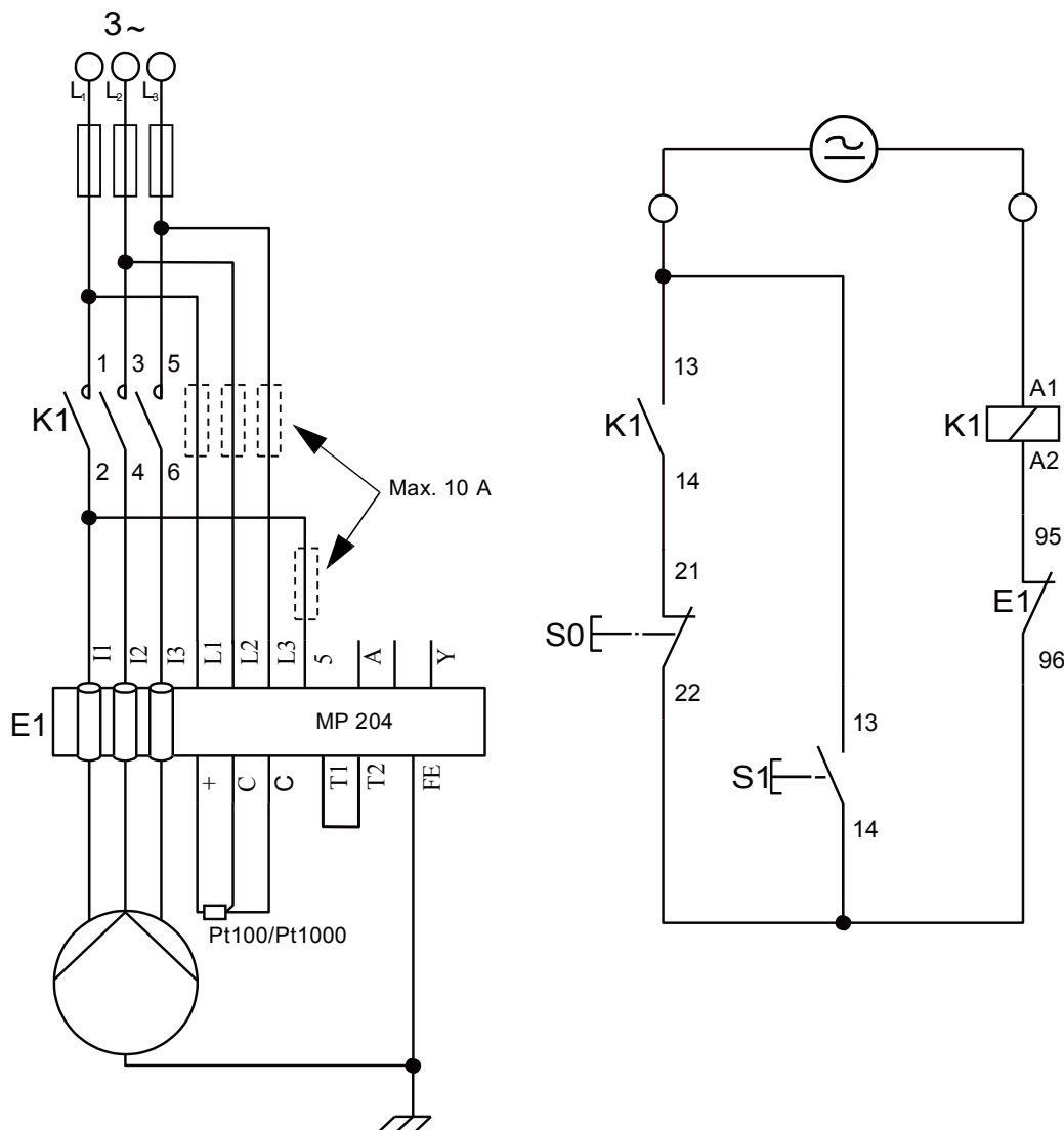
Рис. 120 Трёхфазное соединение
