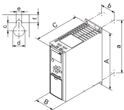
Рис. 106 Корпуса A2 и A3
