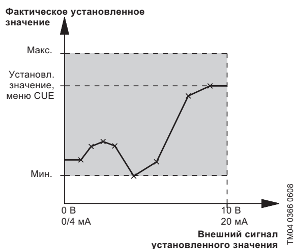
Рис. 79 Внешнее установленное значение по таблице
