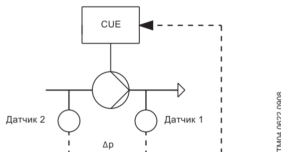
Рис. 91 Перепад давления от двух датчиков
