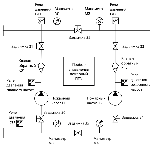
Рис. 57 Примерная гидравлическая схема установки пожаротушения, оснащенной ППУ Control MX
