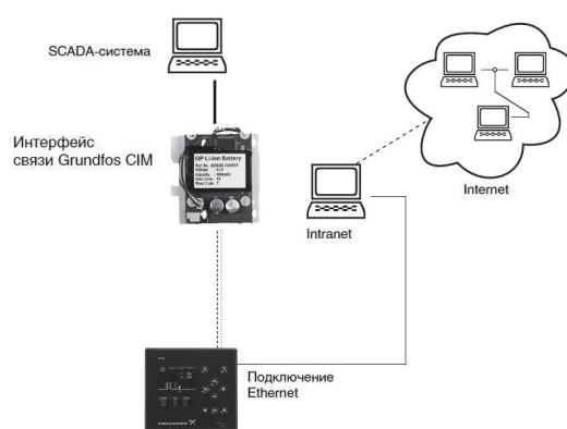
Рис. 41 Передача данных через модуль CIM и локальную сеть
