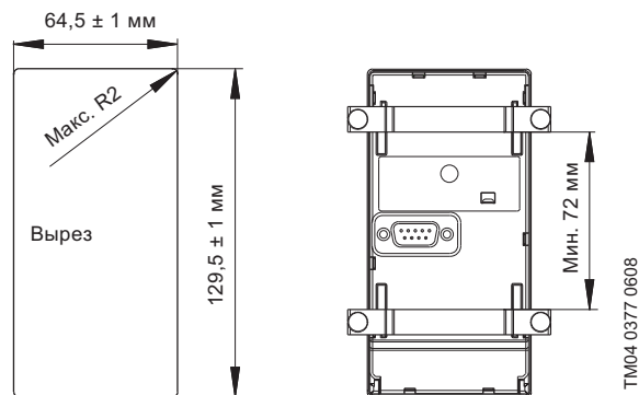
Рис. 114 Монтаж шкафа, размеры выреза
