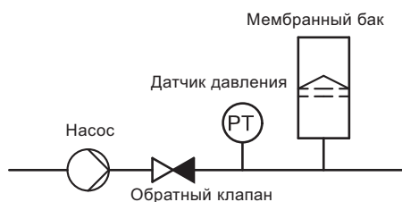
Рис. 83 Расположение обратного клапана и датчика давления в системе, имеющей подпор на входе
