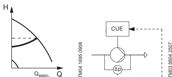
Рис. 89 Перепад давления, параболическая кривая
