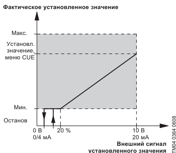
Рис. 78 Внешнее установленное значение с функцией останова
