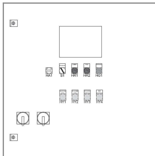
Рис. 59 Прибор управления пожарный. Внешний вид.
