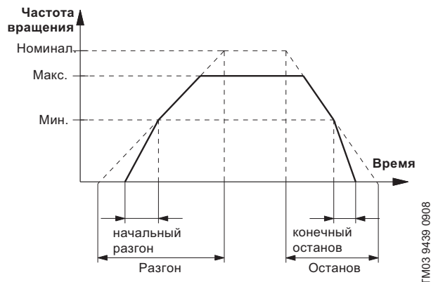
Рис. 88 Разгон и останов CUE
