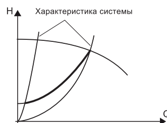
Рис. 15 Характеристика циркуляционной системы
