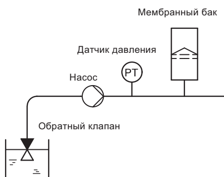
Рис. 82 Расположение обратного клапана и датчика давления в системе, предусматривающей всасывание или работу с отрицательным давлением на входе
