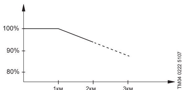
Рис. 105 Снижение тока на выходе при низком атмосферном давлении
