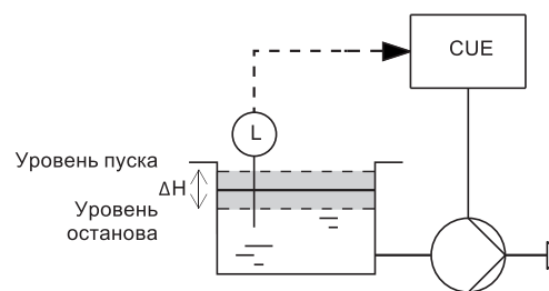
Рис. 84 Постоянный уровень с функцией останова. Разница между значениями уровня срабатывания на пуск и останов
