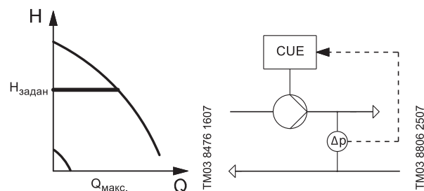
Рис. 65 Постоянный перепад давления в системе
