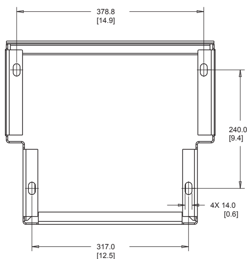
Рис. 115 Шаблон для сверления под цоколь D2h (мм)
