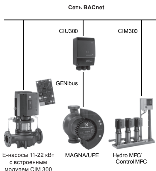
Рис. 140 Модуль CIM/CIU 300 в сети BACnet
