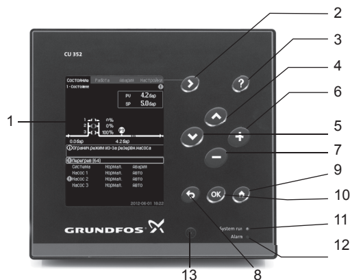
Рис. 19 Панель управления
